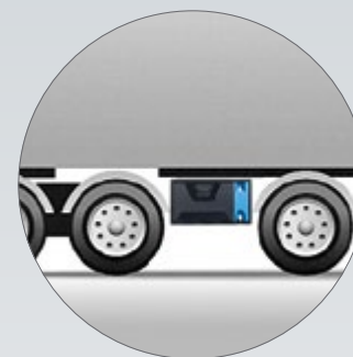
PLUS 1 Normativa ECE R73.01 (L'Omologazione è valida solo con i supporti Co.Par.)
